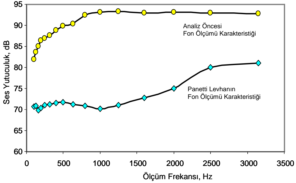
Şekil. Deneysel Fon Ölçüm Karakteristiği
