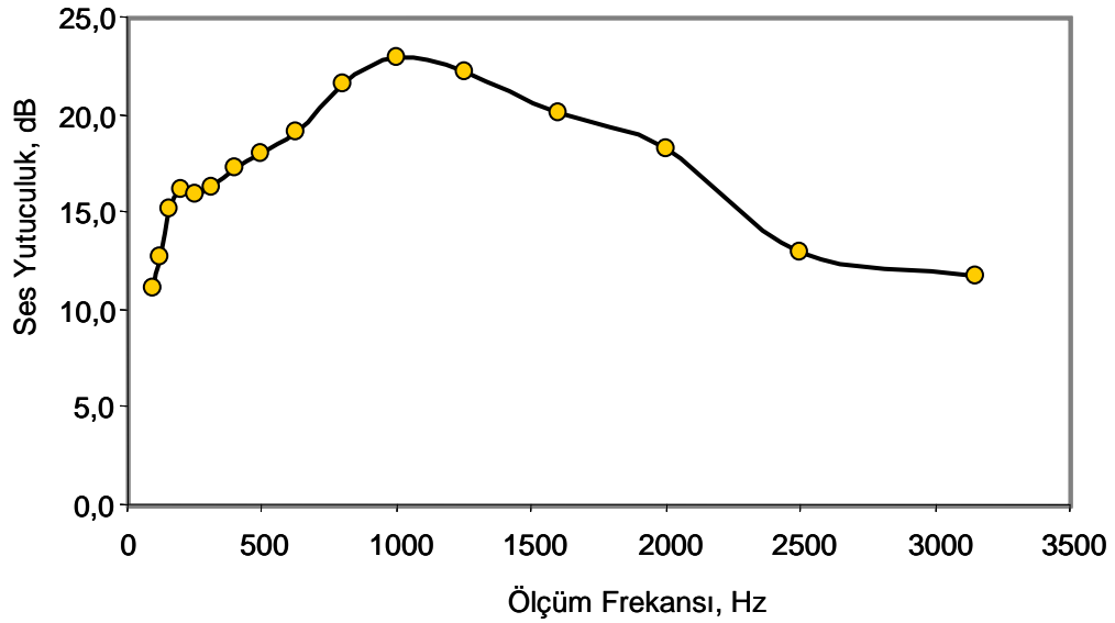
Şekil. Panetti Levhanın Ses Yutuculuk Karakteristiği
